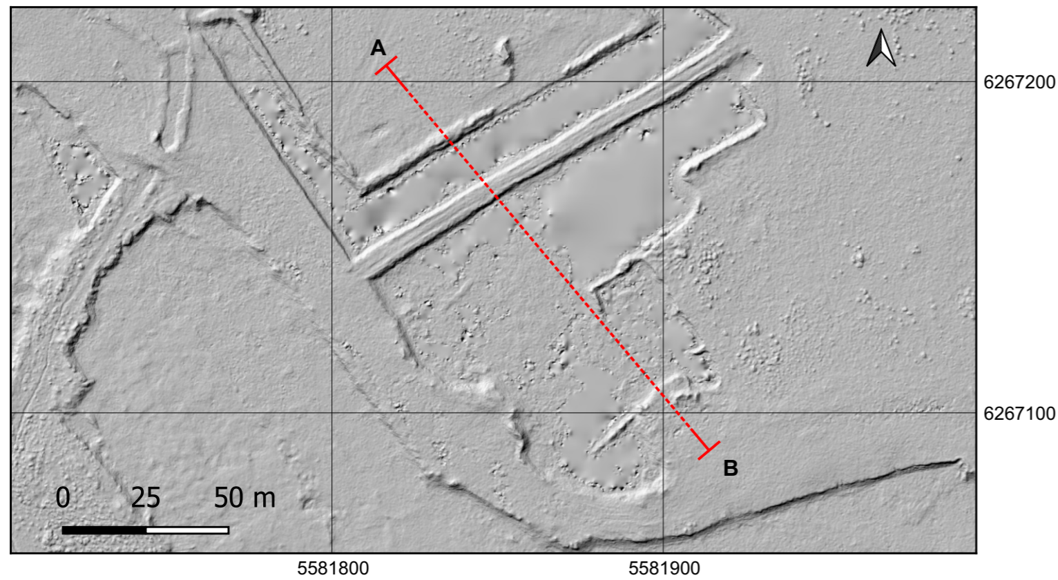
Modelo digital de elevación (mapa de sombras)
