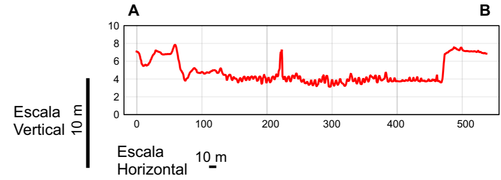
Perfil topográfico sobrealzado
