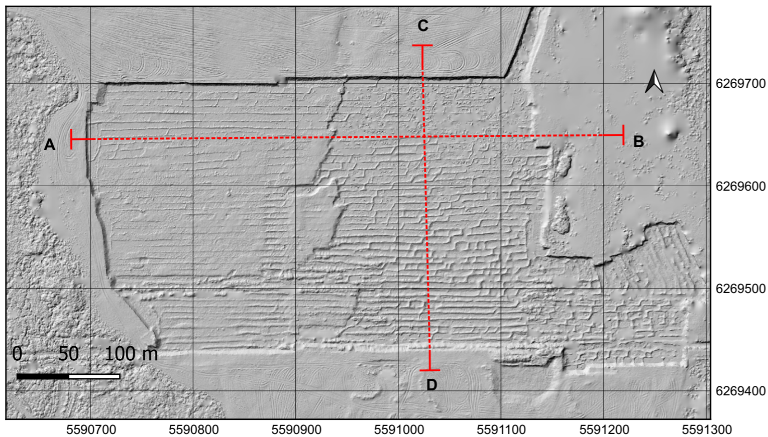
Modelo digital de elevación (mapa de sombras)
