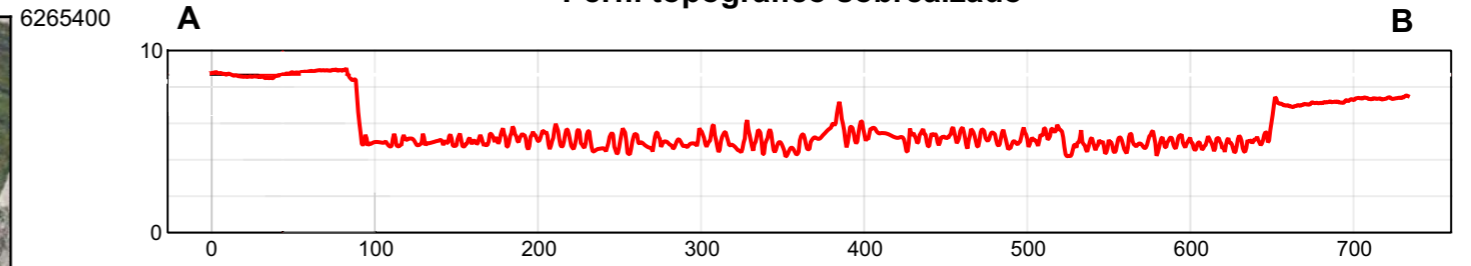
Perfil topográfico sobrealzado
