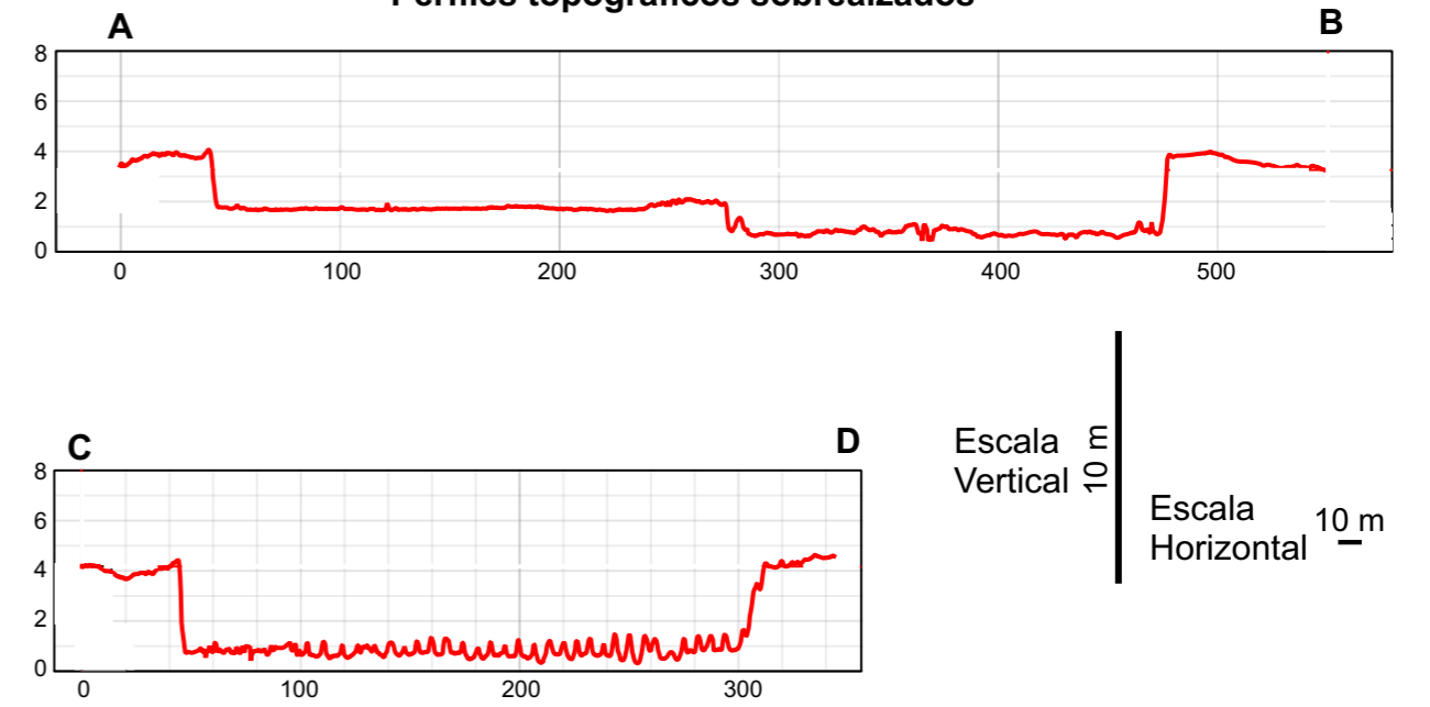
Perfiles topográficos sobrealzados
