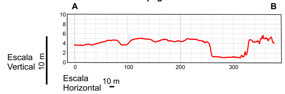
Perfil topográfico sobrealzado
