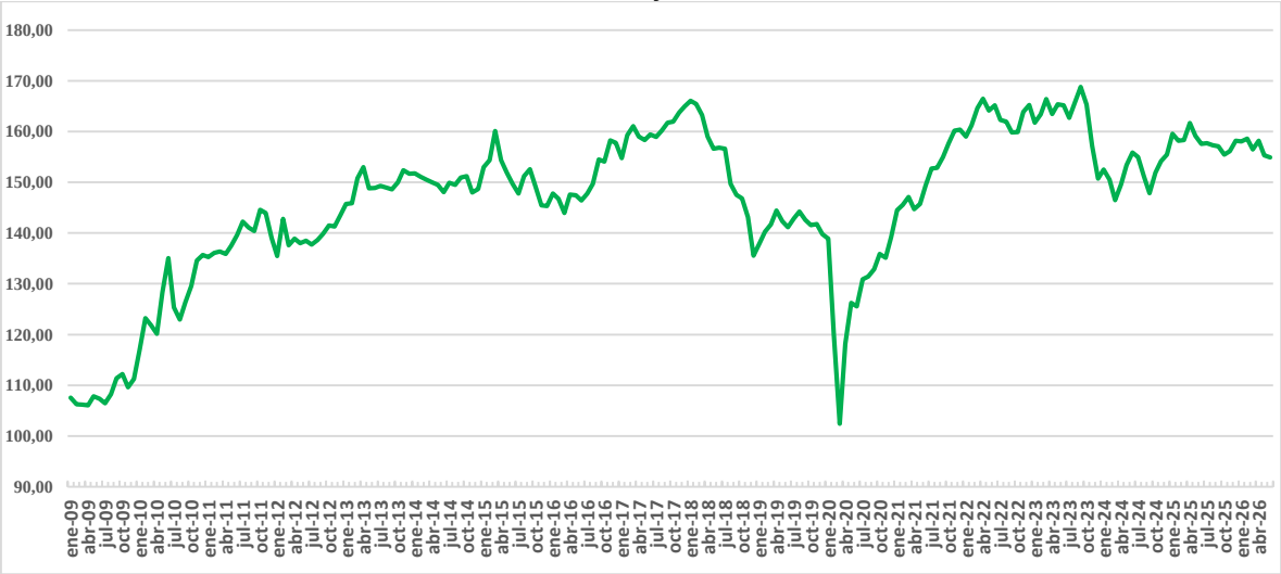
Gráfico 1. Indicador Sintético de Actividad Económica de la provincia de Entre Ríos – ISAEER. Enero 2009 –junio 2026.
