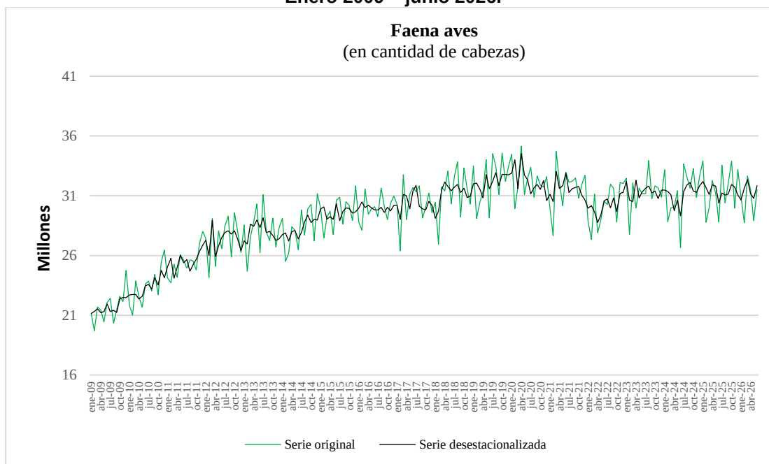
Gráfico 7. Faena de aves, en cantidad de cabezas. Series original y desestacionalizada. Enero 2009 – junio 2026.
