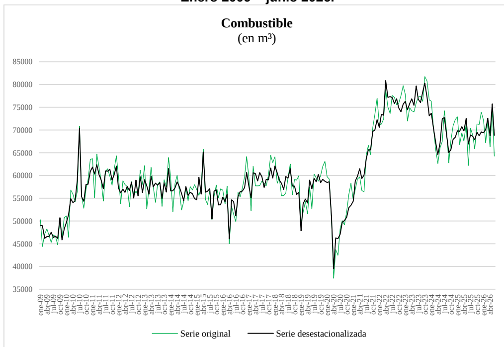
Gráfico 2. Consumo de combustible, en m 3 . Series original y desestacionalizada. Enero 2009 – junio 2026.
