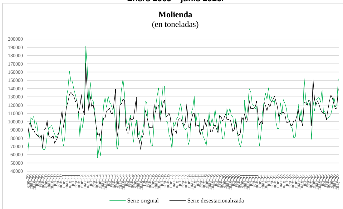
Gráfico 8. Molienda, en toneladas. Series original y desestacionalizada. Enero 2009 – junio 2026.
