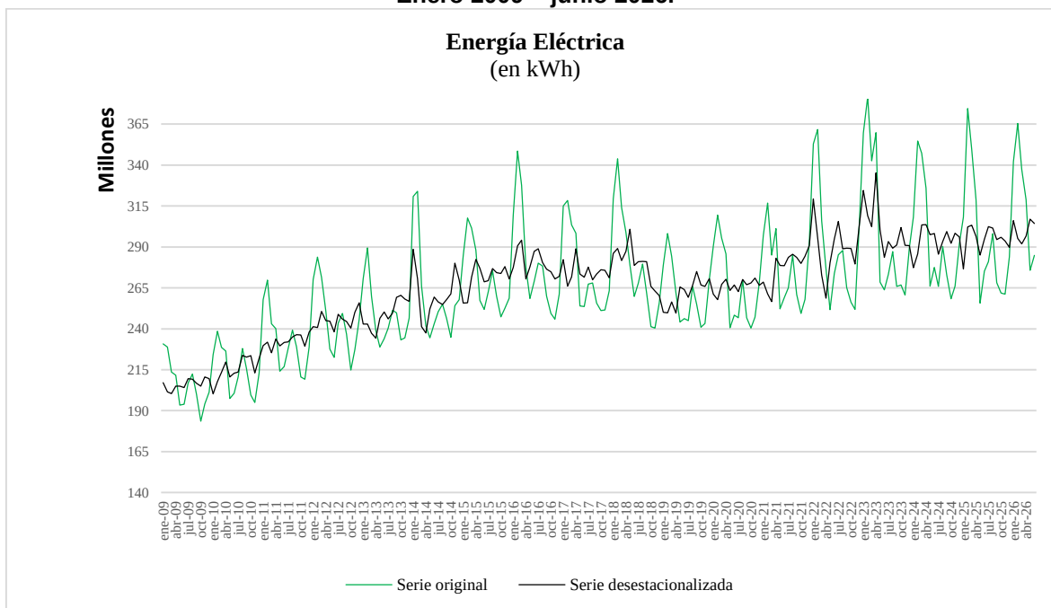
Gráfico 3. Consumo de energía eléctrica, en kWh. Series original y desestacionalizada. Enero 2009 – junio 2026.
