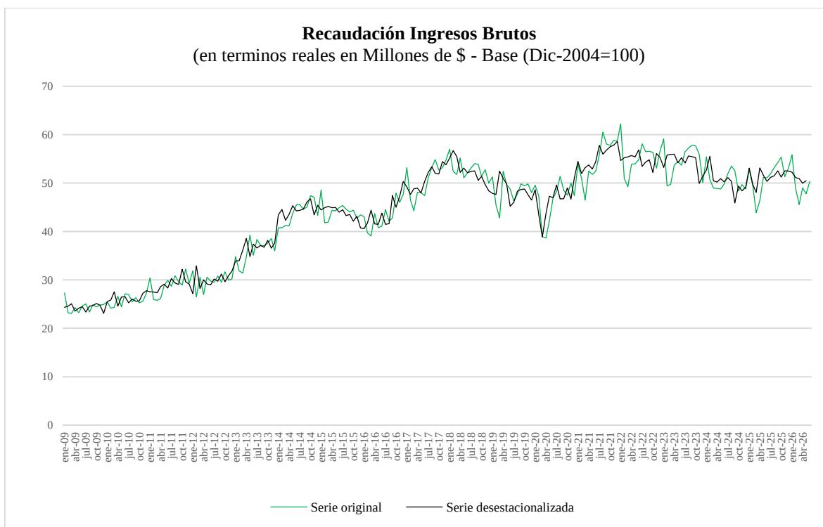
Gráfico 6. Recaudación Ingresos Brutos (en términos reales) en Millones de $, Base Dic-2004=100. Series original y desestacionalizada. Enero 2009 – junio 2026.
