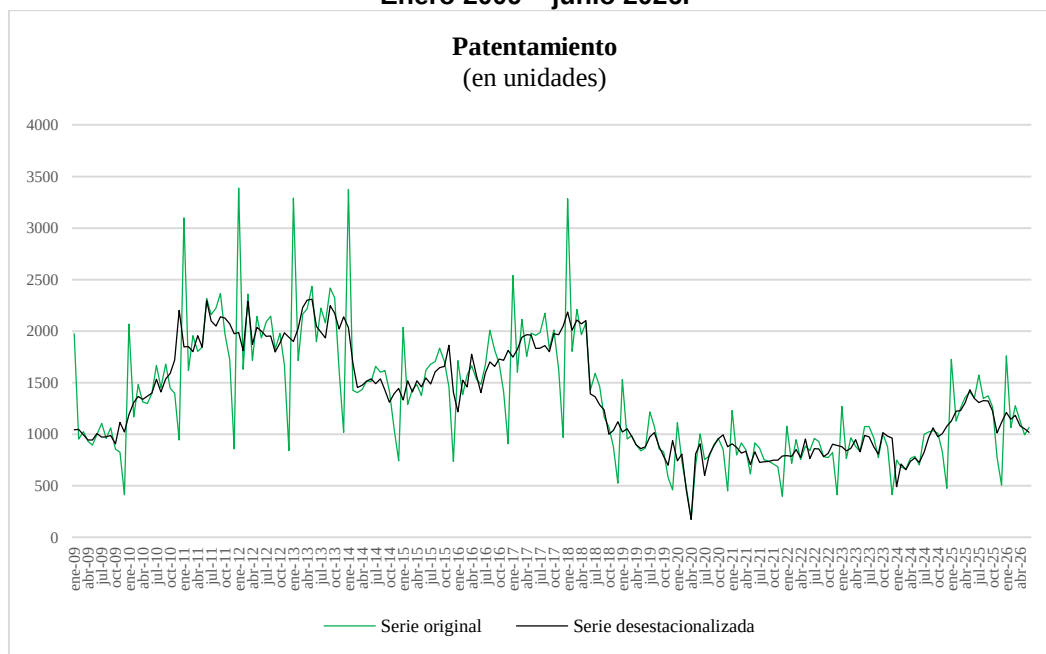
Gráfico 5. Patentamiento de 0 km, en unidades. Series original y desestacionalizada. Enero 2009 – junio 2026.
