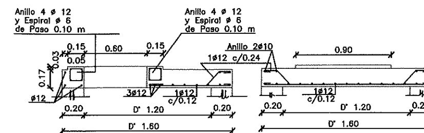
Corte por A - A
