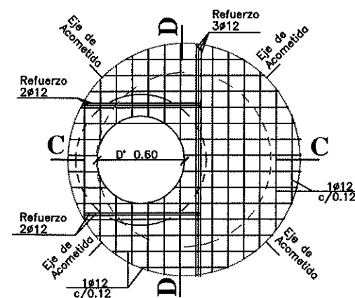
Planta por F - F
