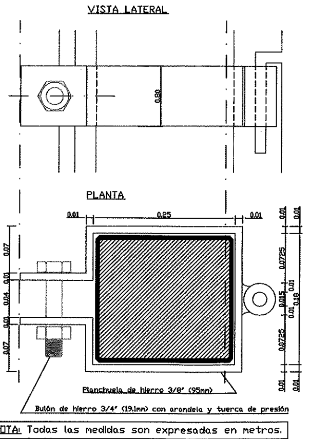
DETALLE N° 1 Bisagra portón sin escala
