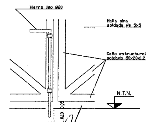
DETALLE N° 2 Traba de portón sin escala
