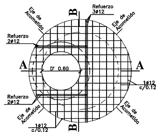
Planta por E - E
