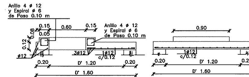
Corte por C - C
