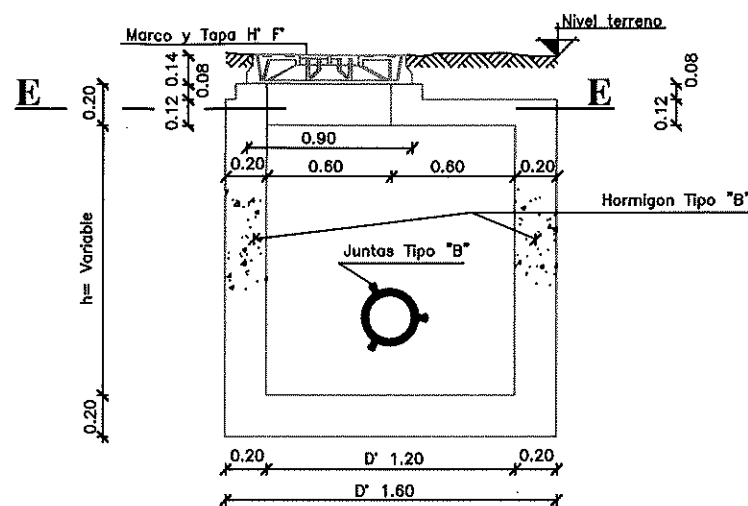
Corte por C - C
