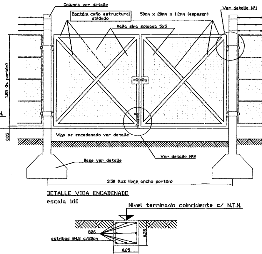
VISTA FRENTE PORTON escala 1:20
