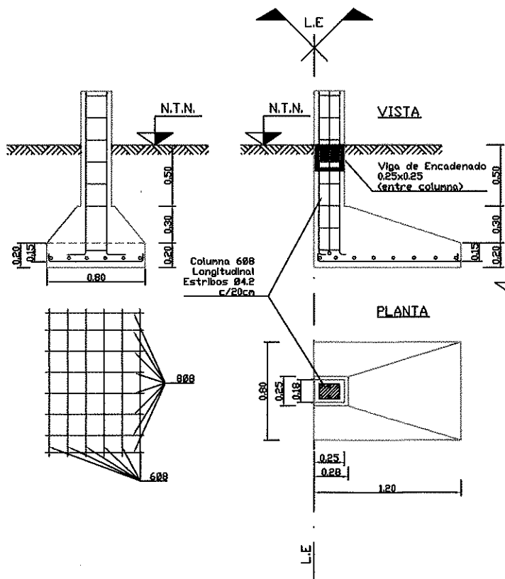
DETALLE DE ESTRUCTURA escala 1:20
