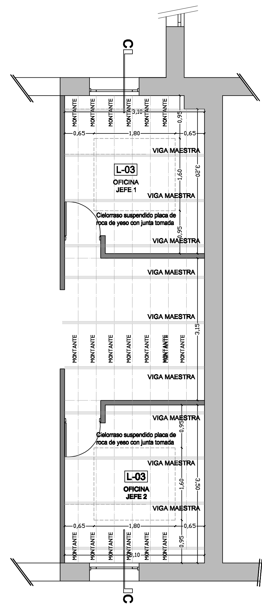
PLANTA - Cielorraso Superior
