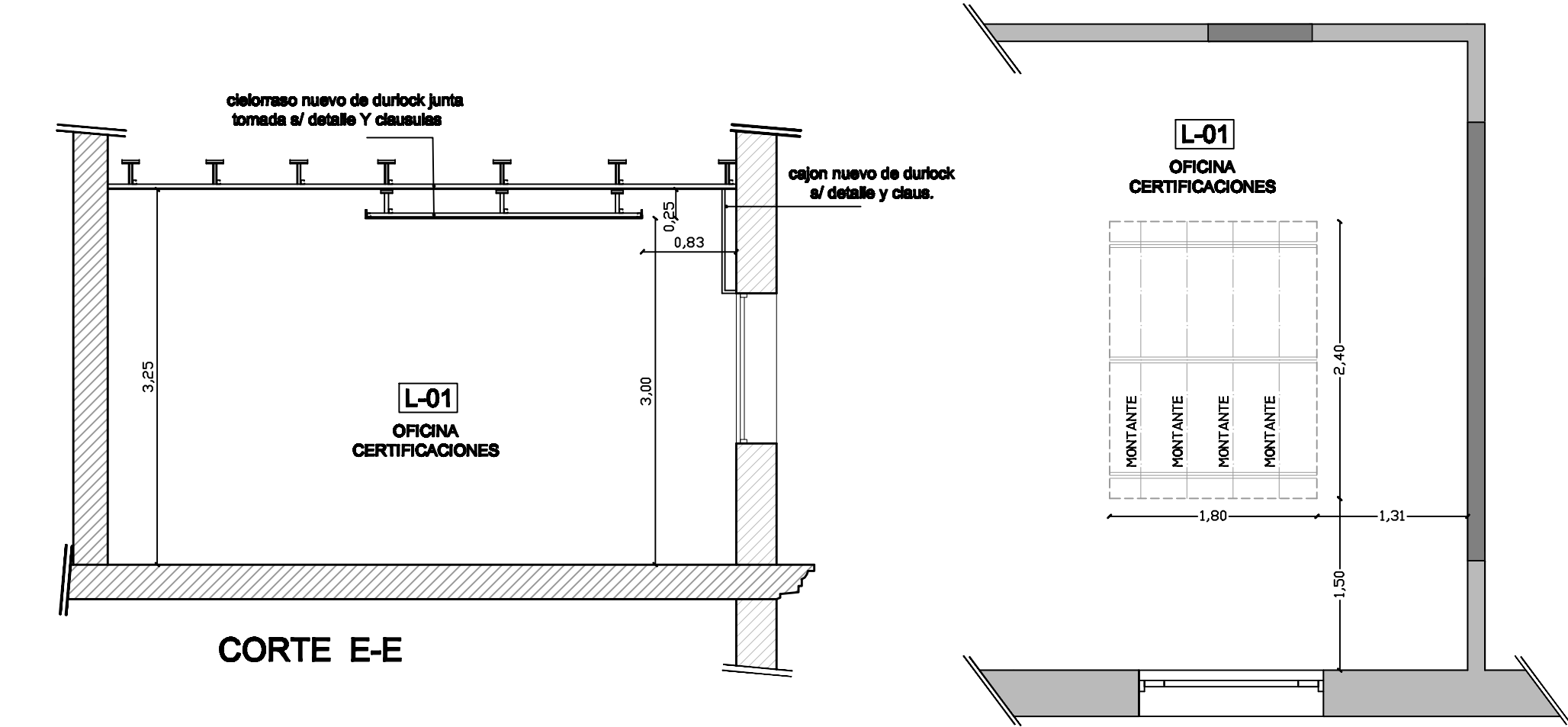
PLANTA - Cieloraso Inferior (bandeja)
