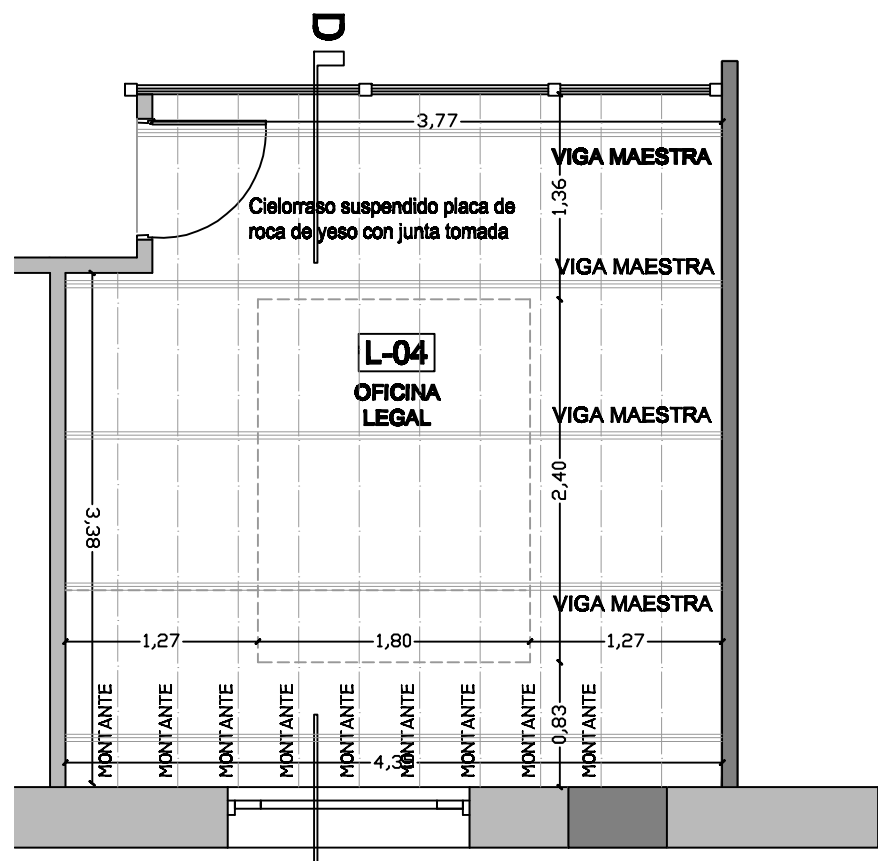
PLANTA - Cieloraso Superior
