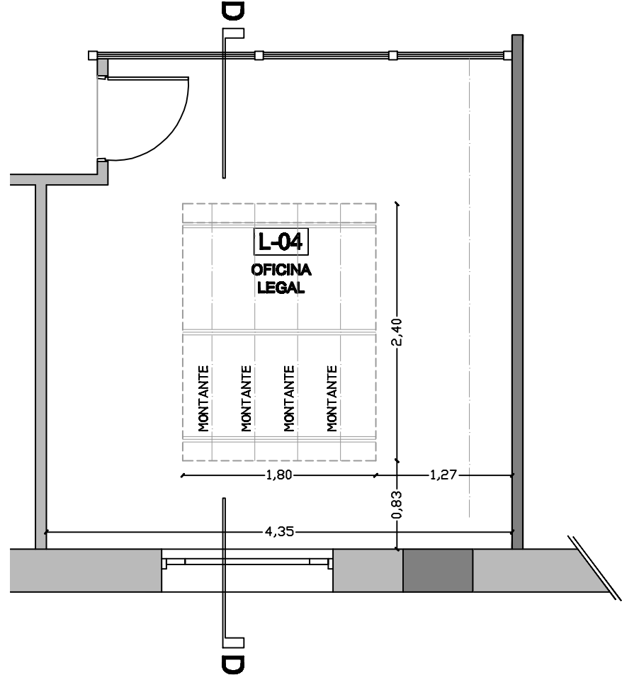
PLANTA - Cieloraso Inferior (bandeja)
