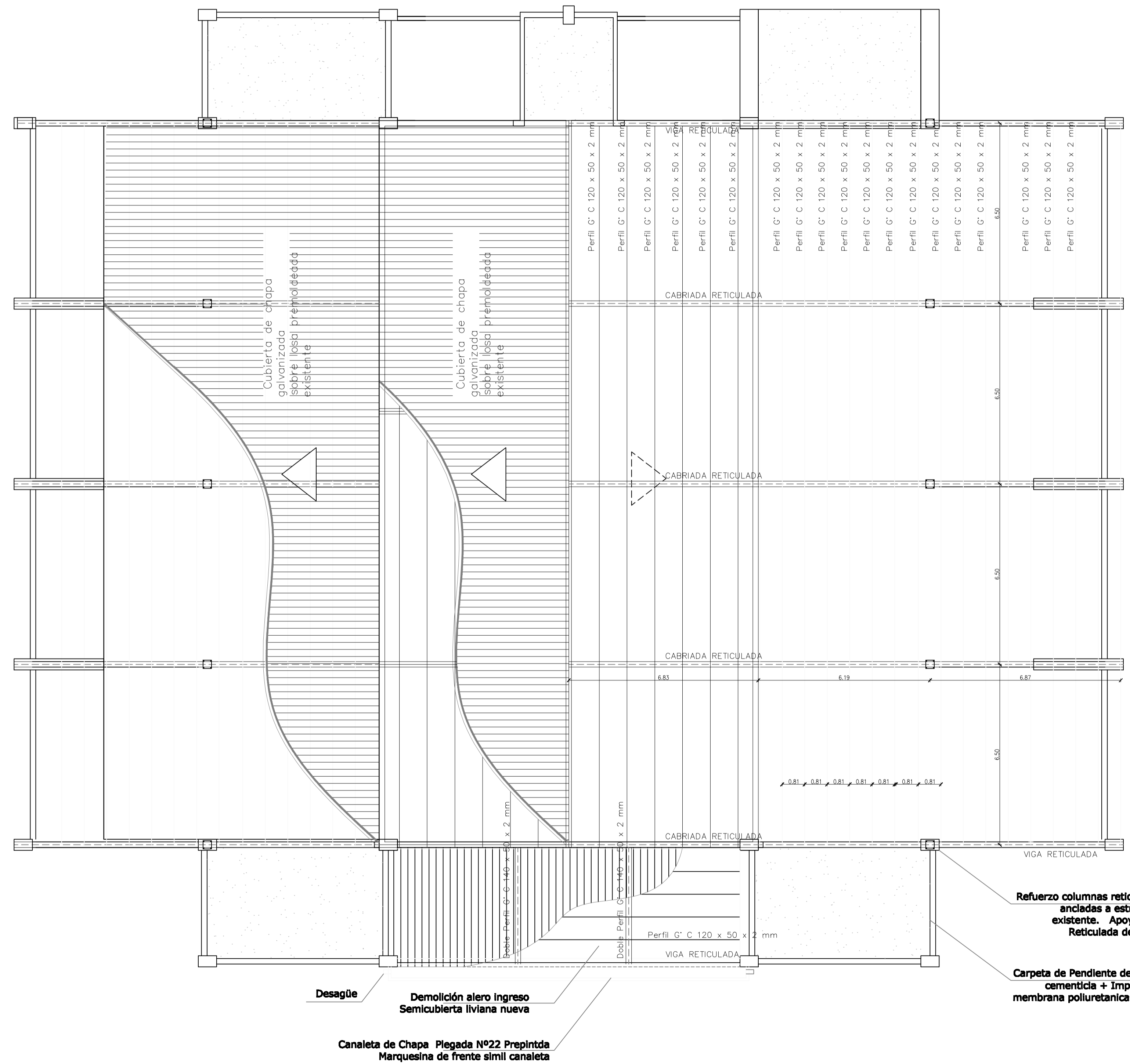
PLANTA de ESTRUCTURA DE TECHOS NUEVOS
