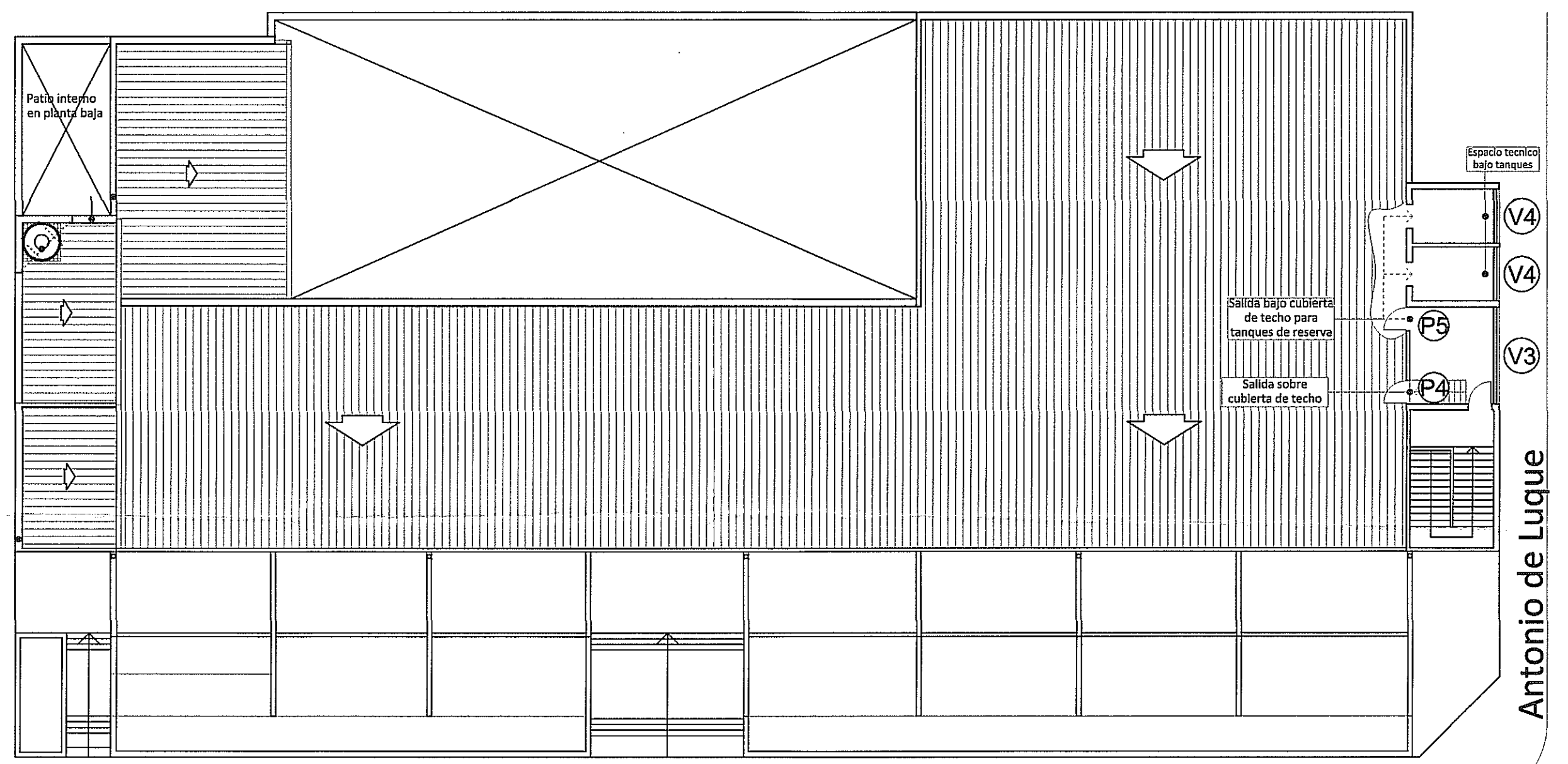
Planta de techo
