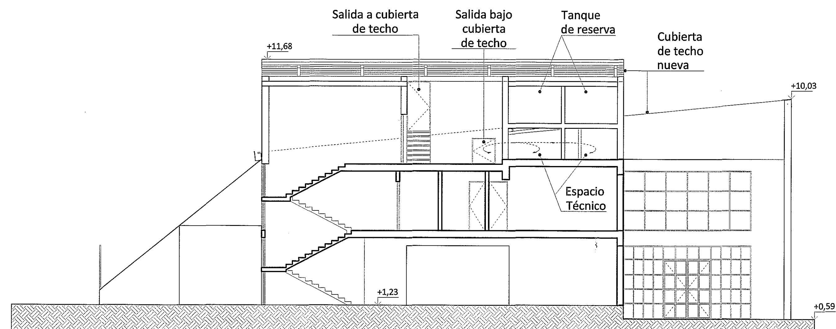
Corte 1:1
