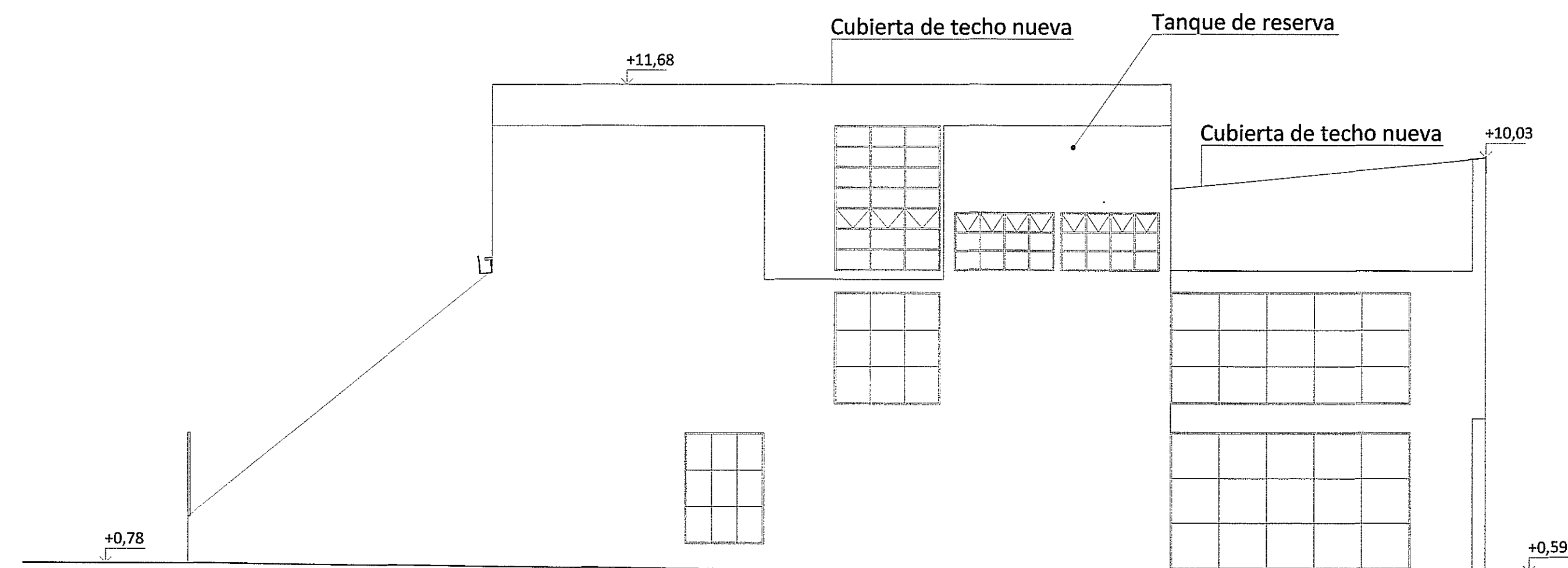
Fachada Sur
