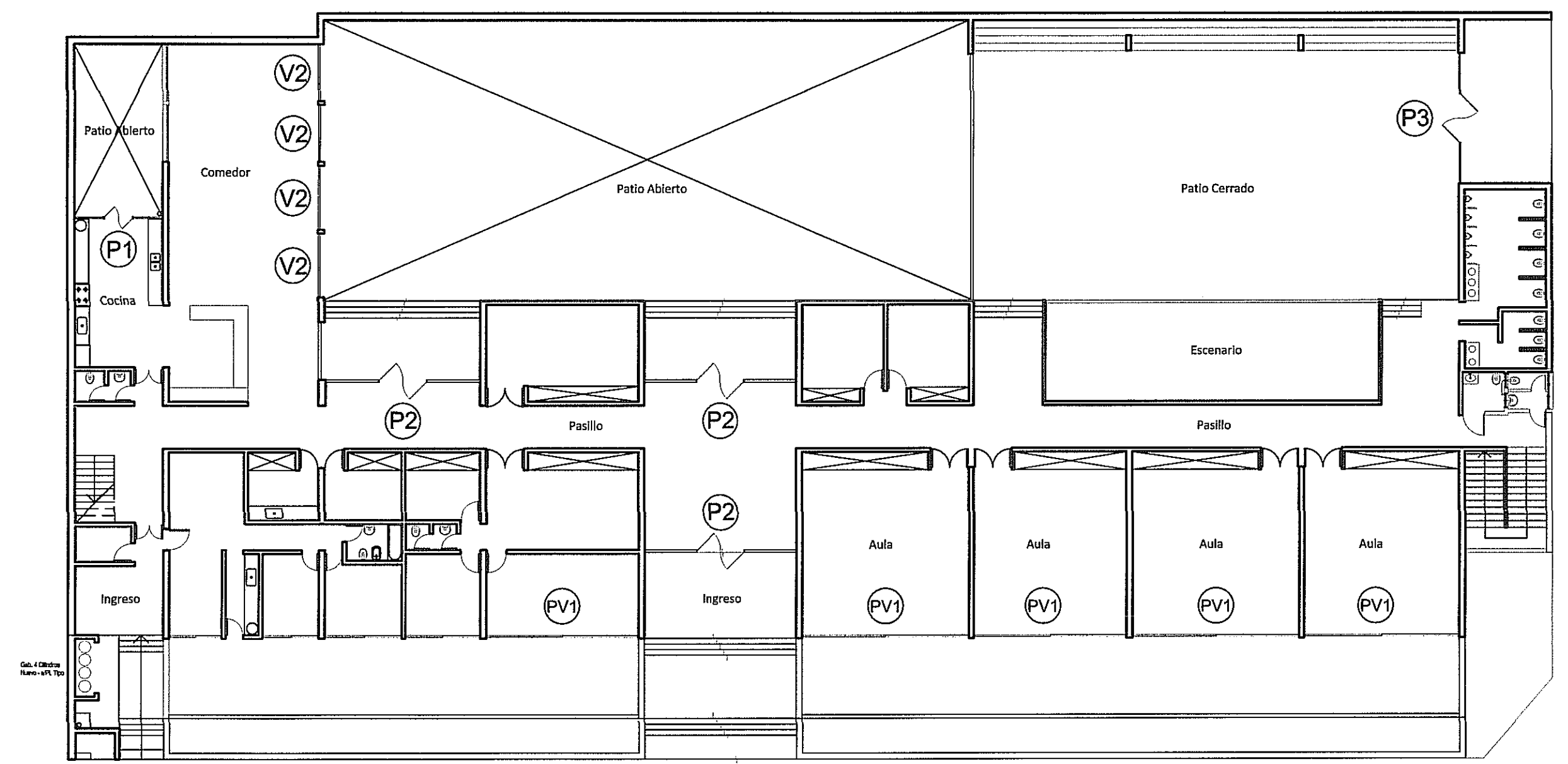
Planta baja
