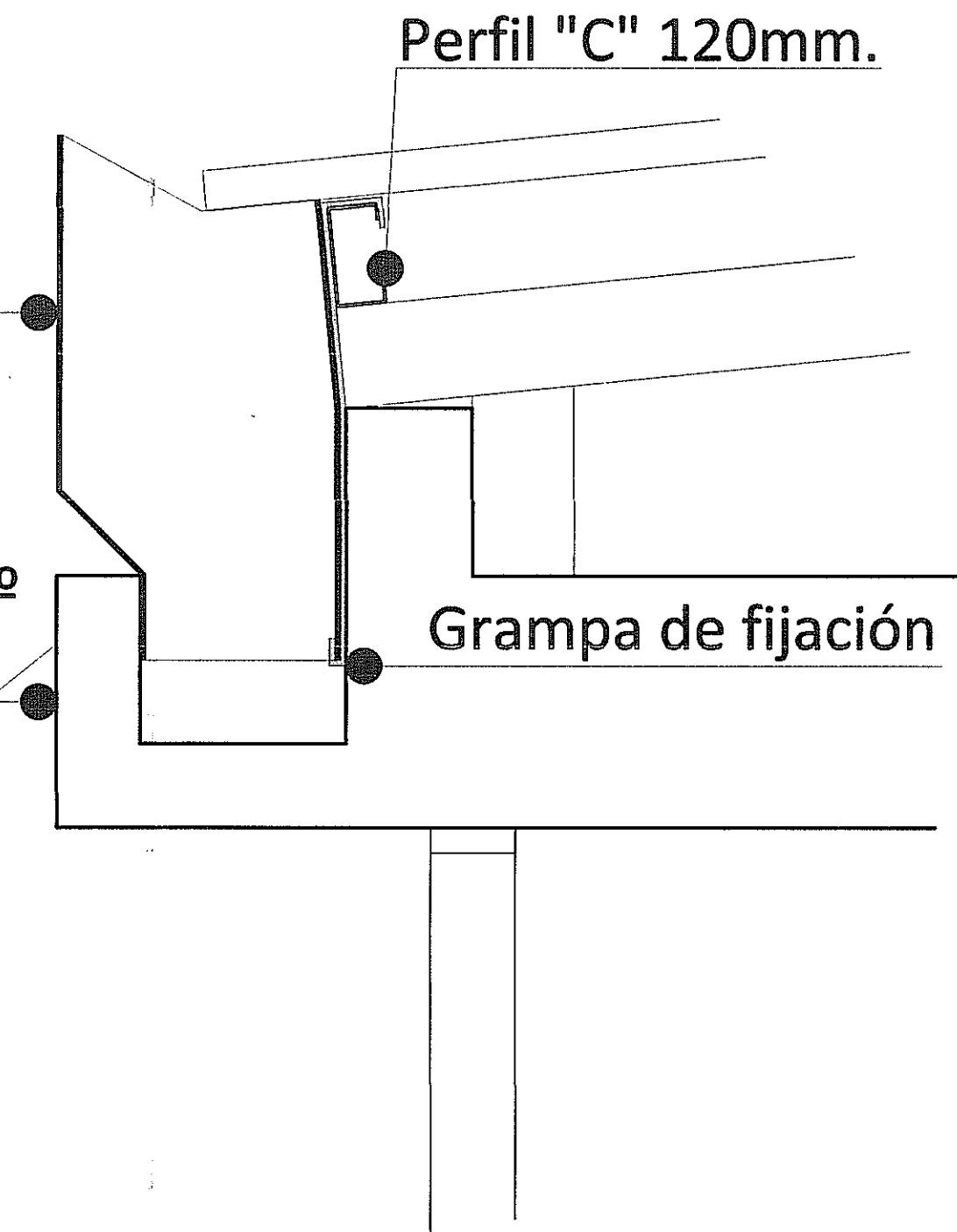
Corte
