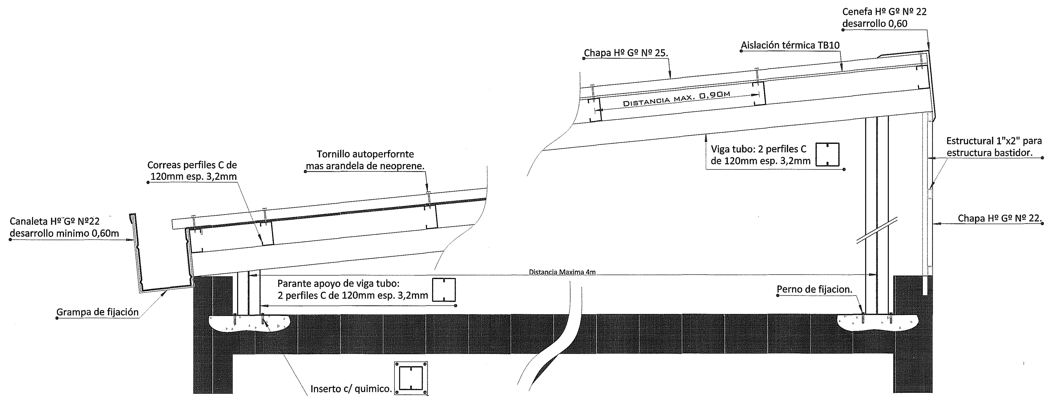
Detalle 2
