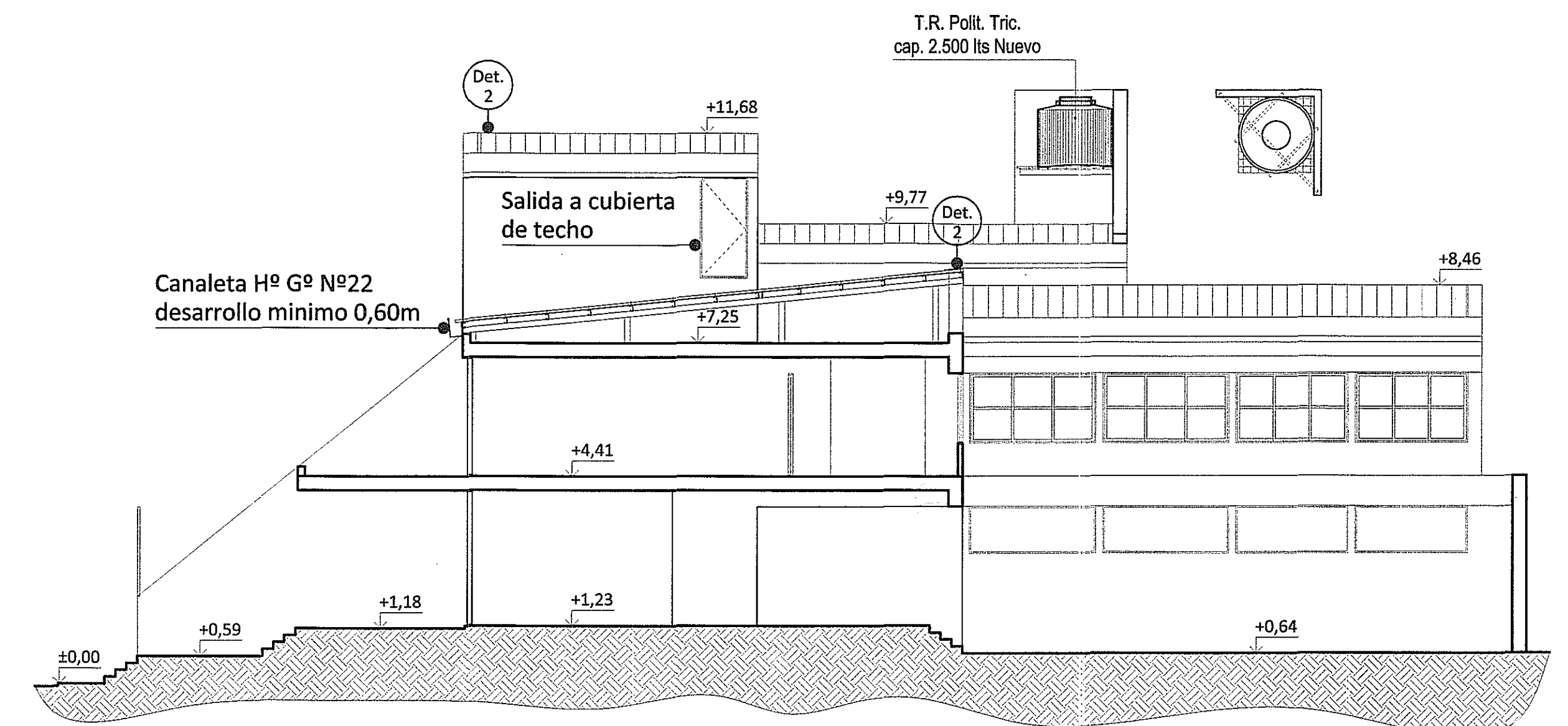
Corte 3:3
