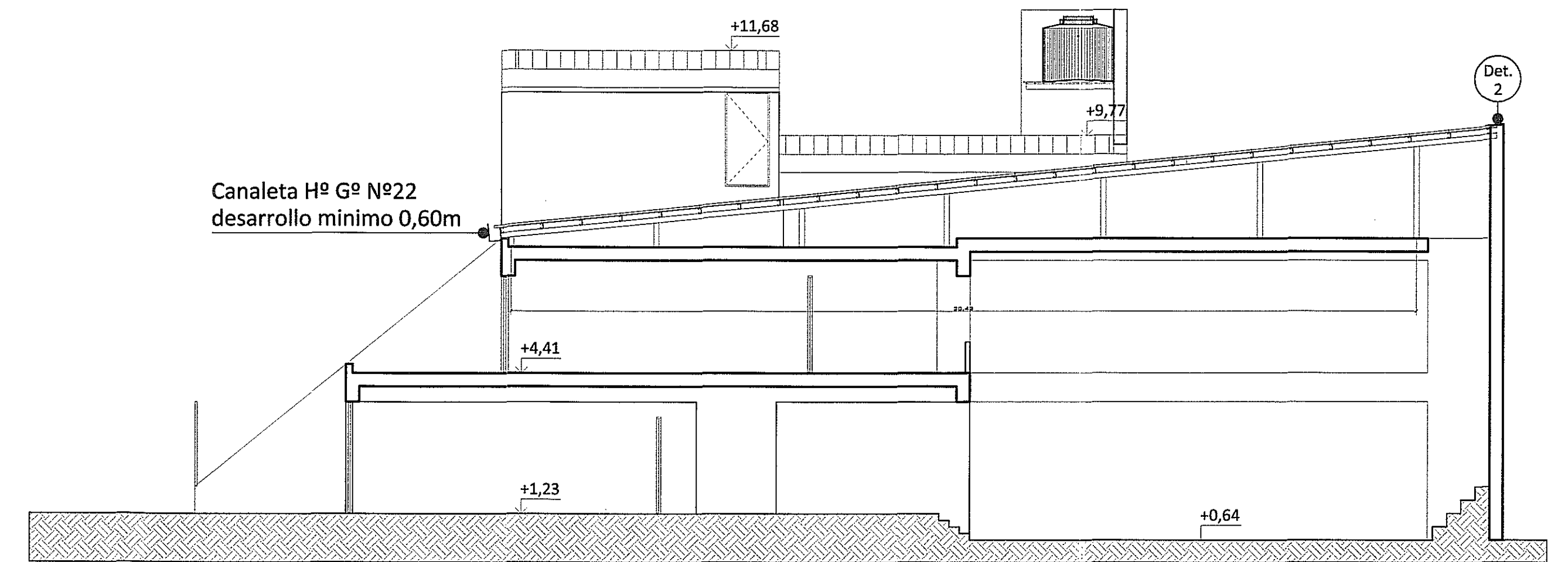
Corte 2:2
