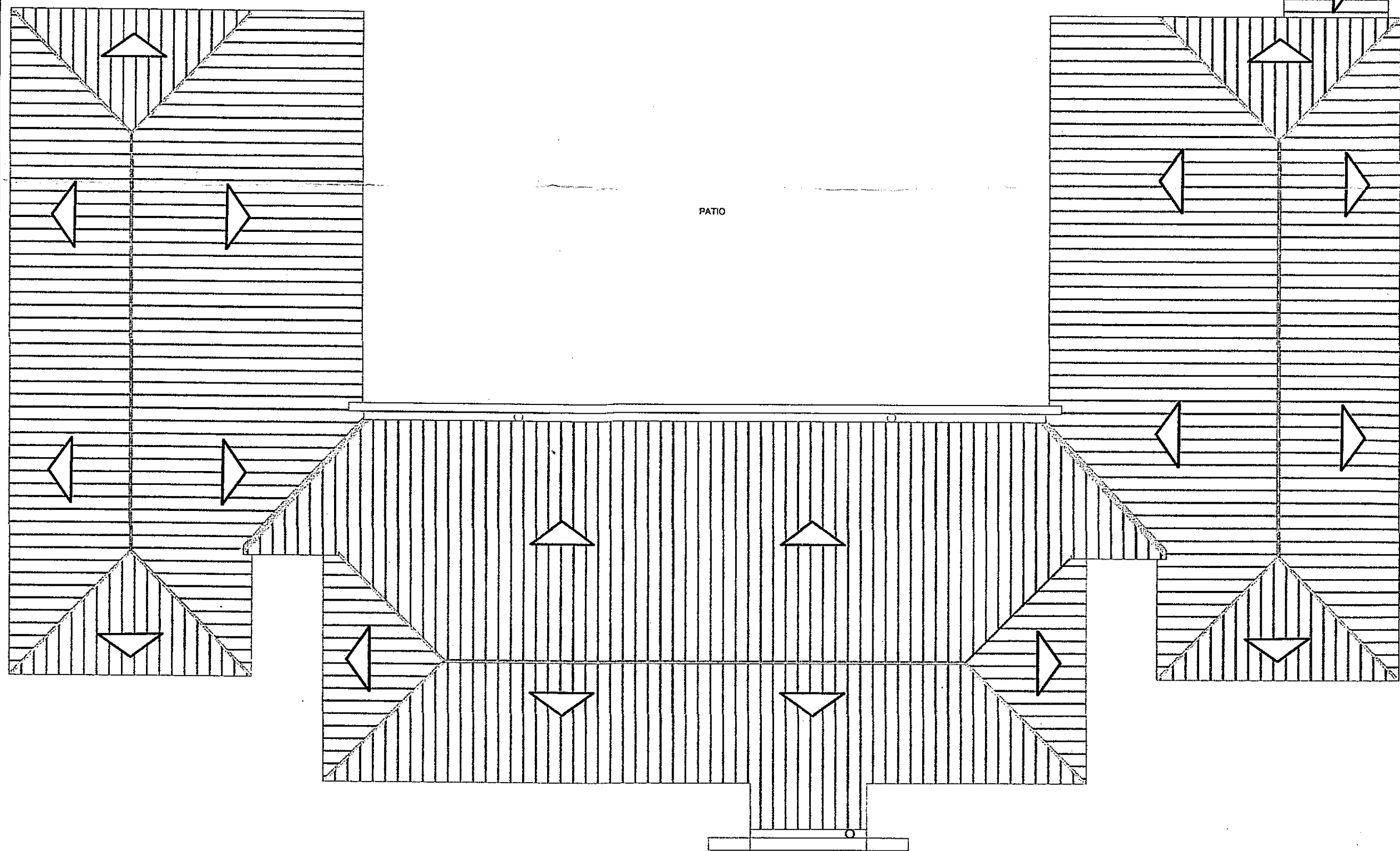
PLANTA TECHO
