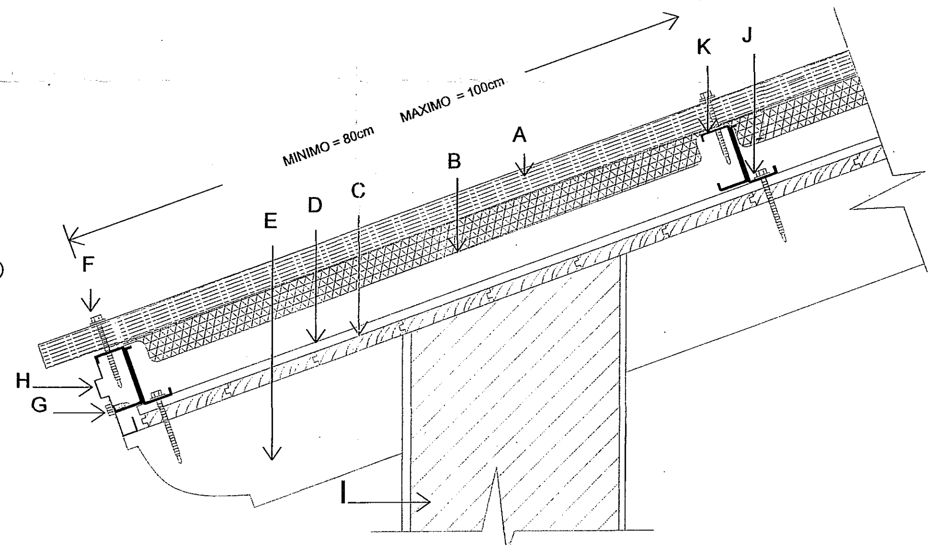
DETALLE 1 Escala 1:10
