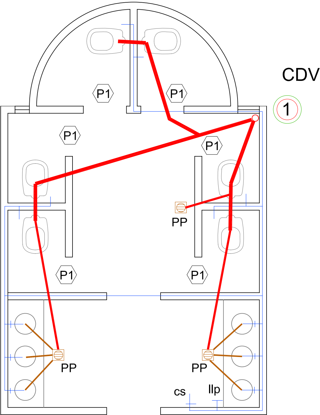
Tipo 3 Planta Alta Cant. 2
