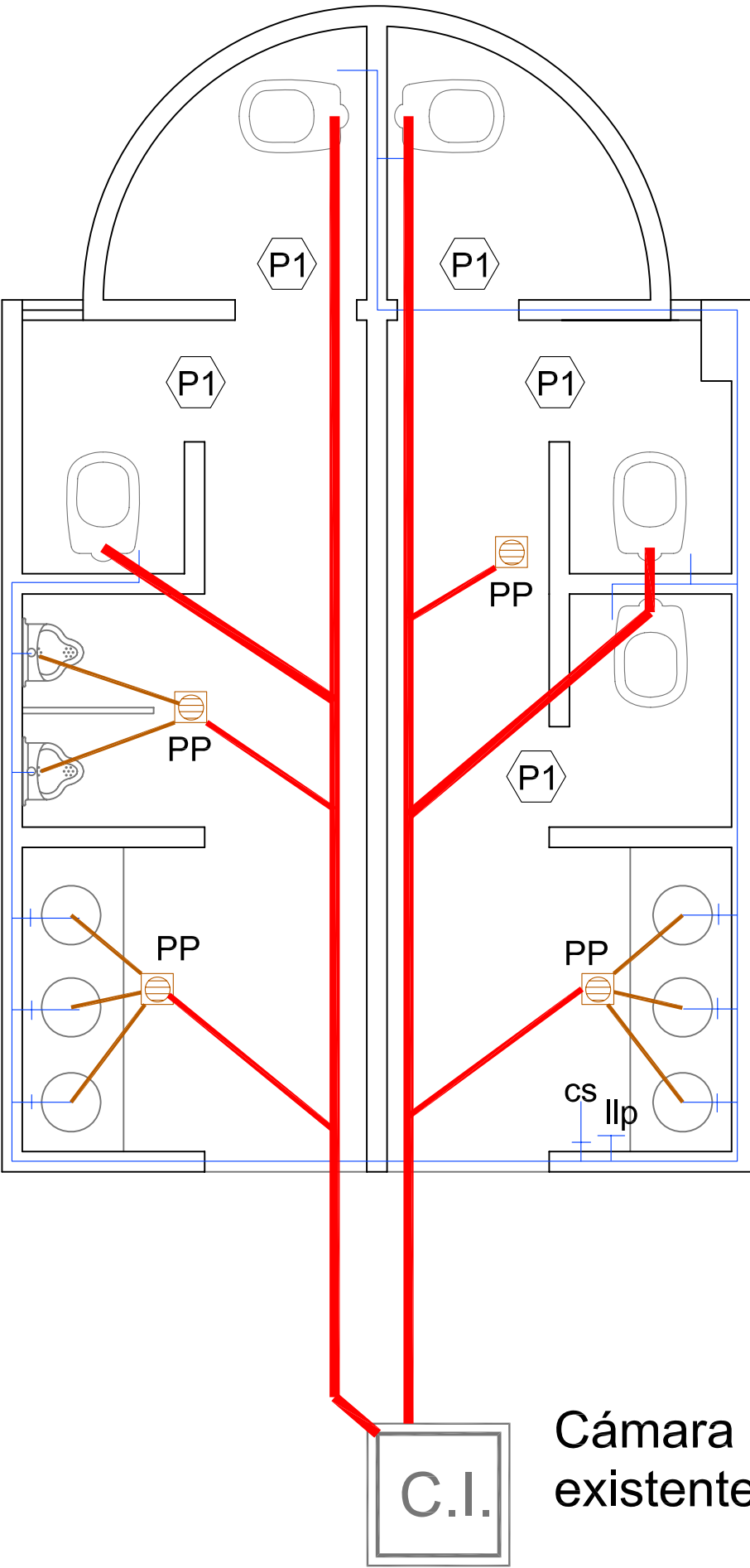
Tipo 1 Planta Baja Cant. 4
