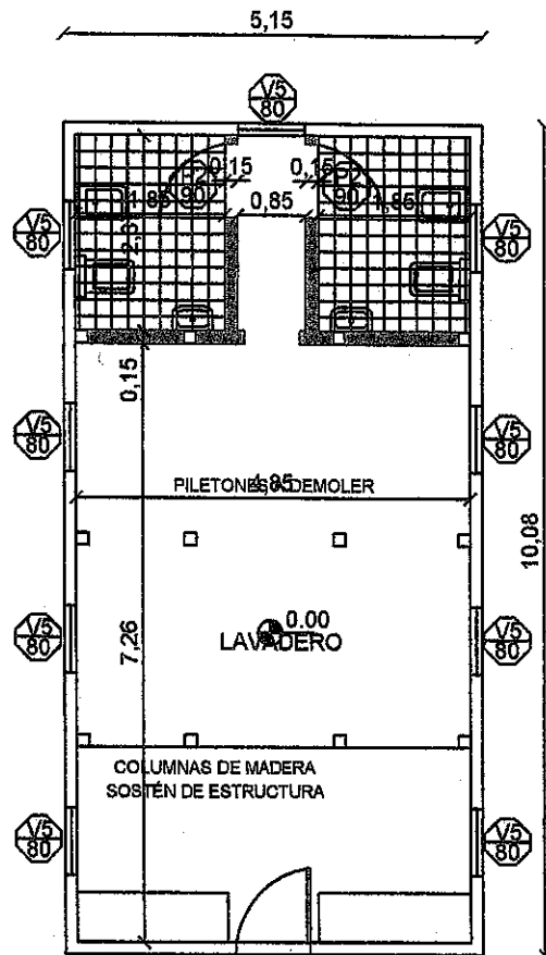
PLANTA
