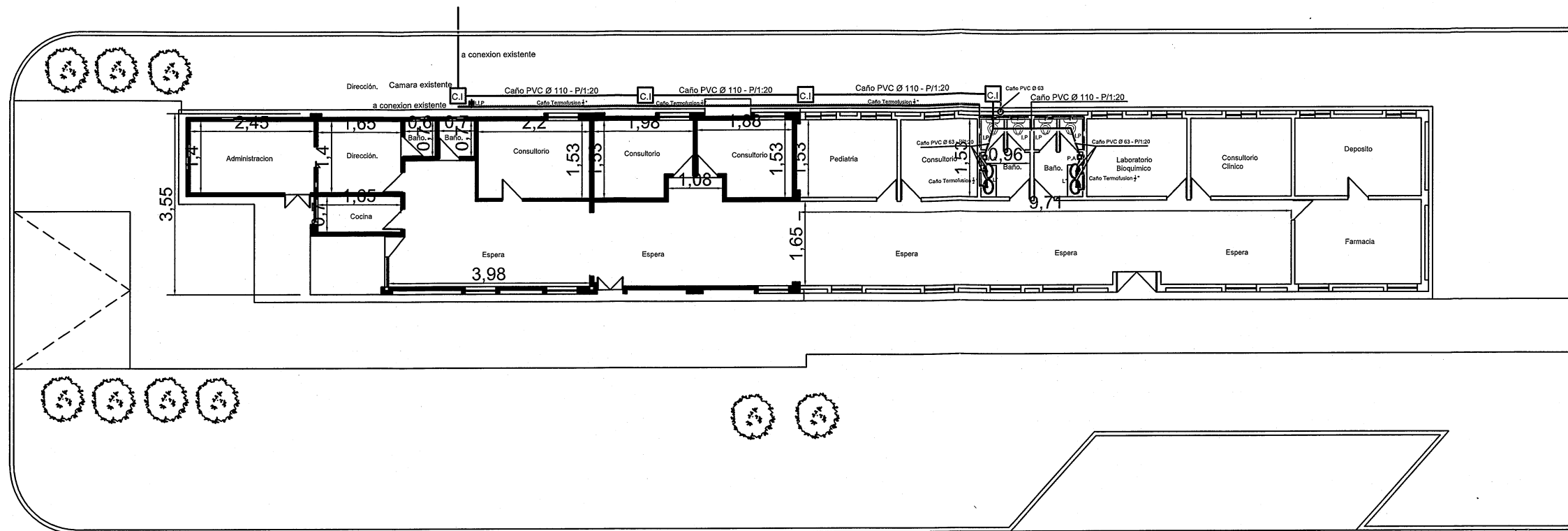
PLANTA INST. SANITARIA
