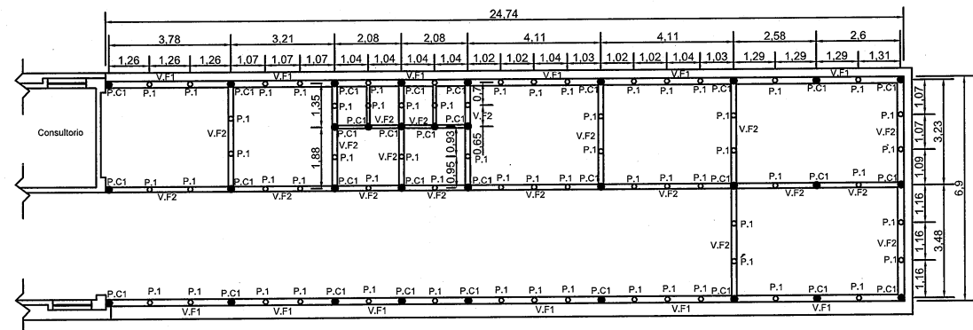
PLANTA DE FUNDACIONES
