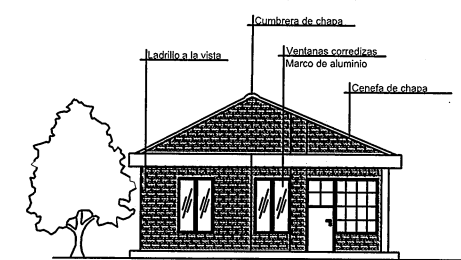
FACHADA
