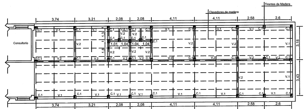
PLANTA DE ESTRUCTURA
