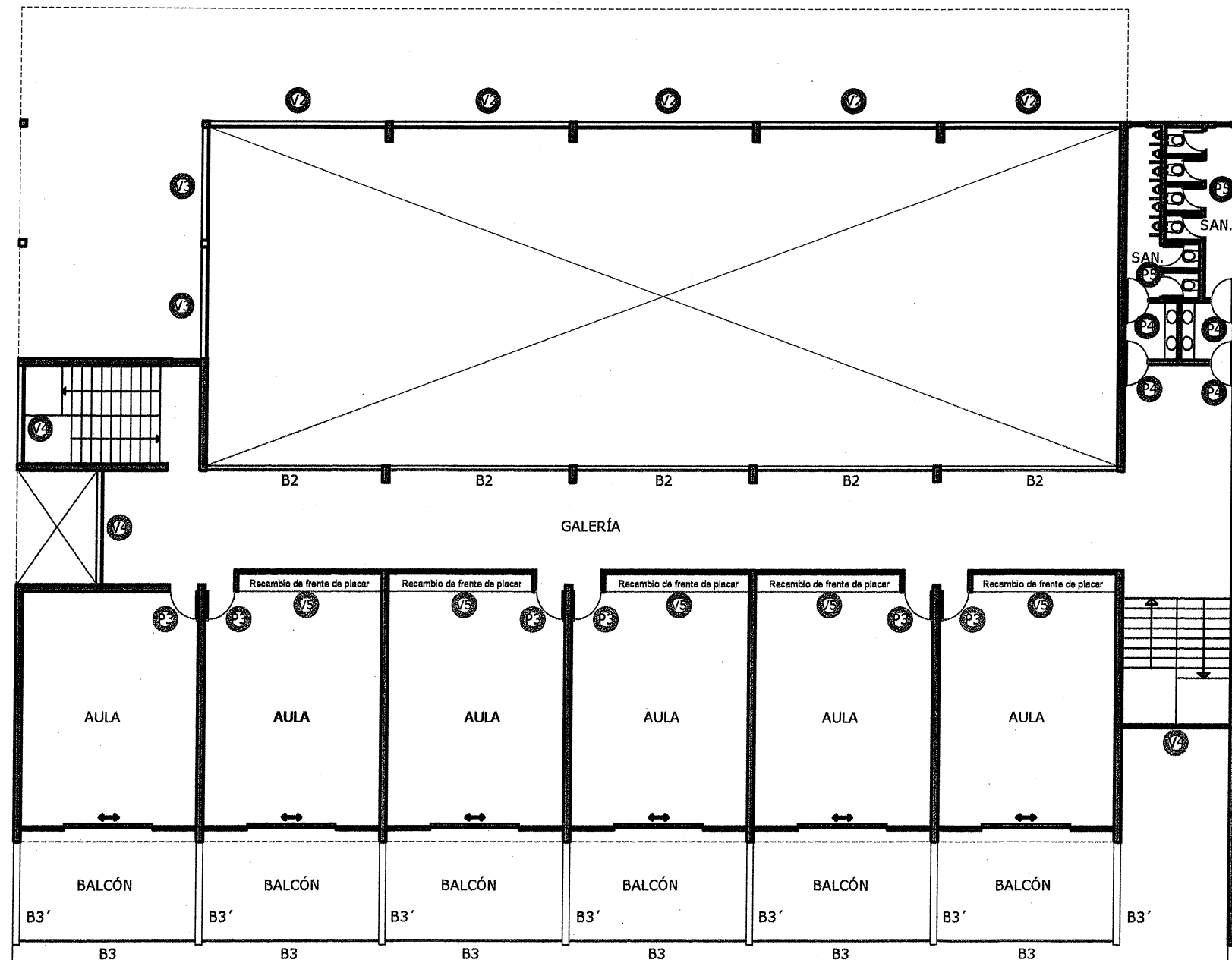
PRIMER PISO
