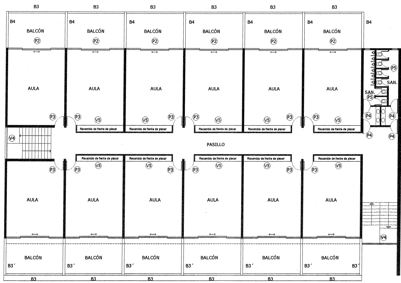
SEGUNDO PISO
