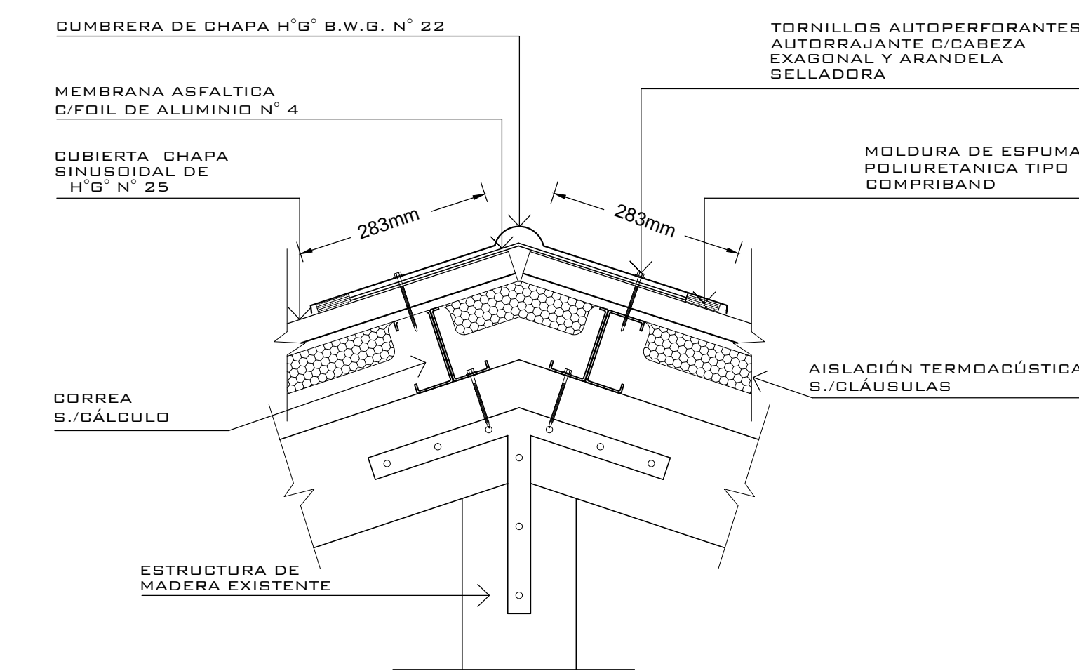
DETALLE DE CUMBRERA (1:5)
