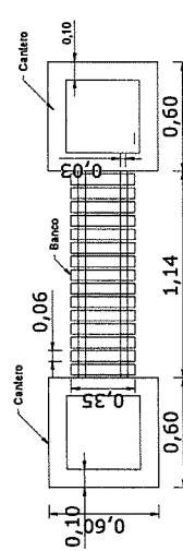
Planta
